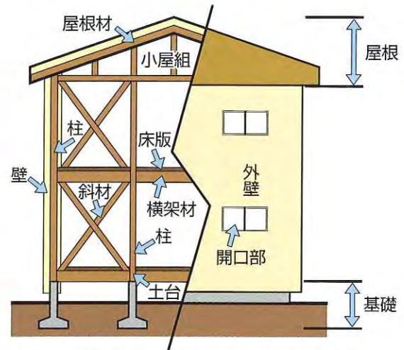
木造(在来軸組工法)の戸建住宅の例
