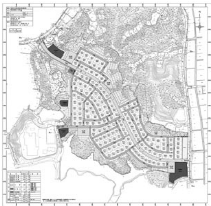
変更された犀川住宅団地計画図
